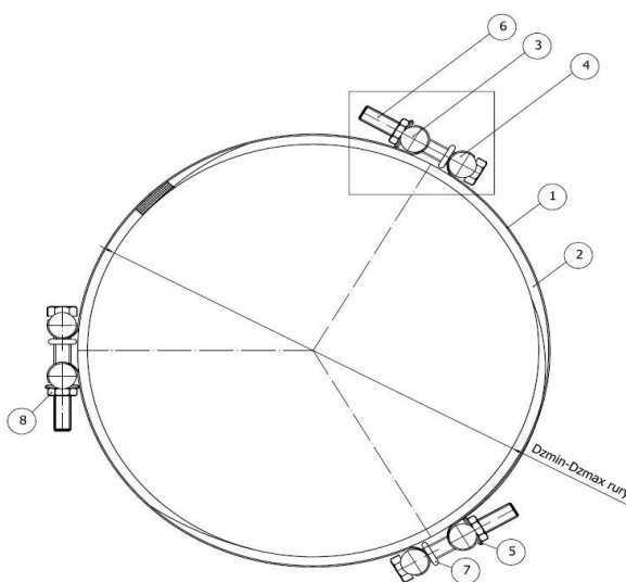
Opaska połączeniowa dwudzielna z uziemieniem
