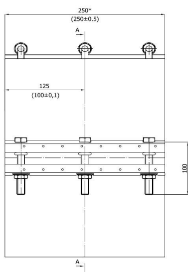
Opaska połączeniowa dwudzielna z uziemieniem
