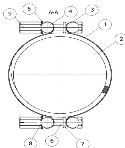
Opaska połączeniowa dwudzielna z uziemieniem
